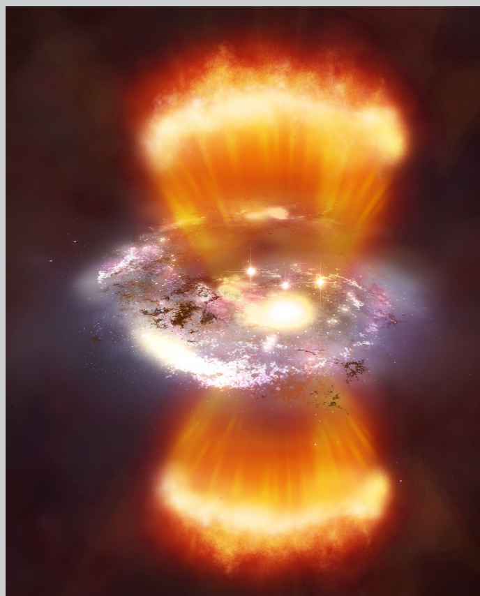
Astrofyzika
